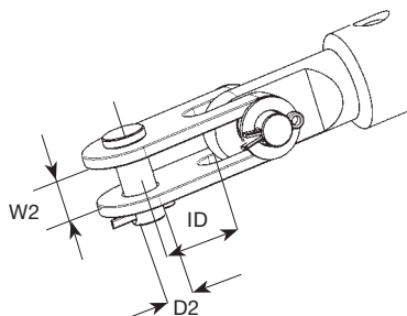
Furlex standardtoggel.
