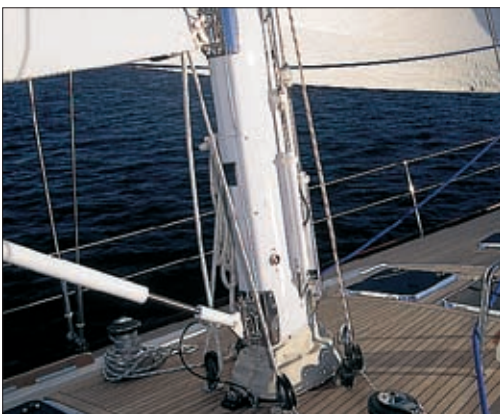
Hydraulique Seldén intégrée. Tous les composants hydrauliques sont à l'intérieur du mât.
