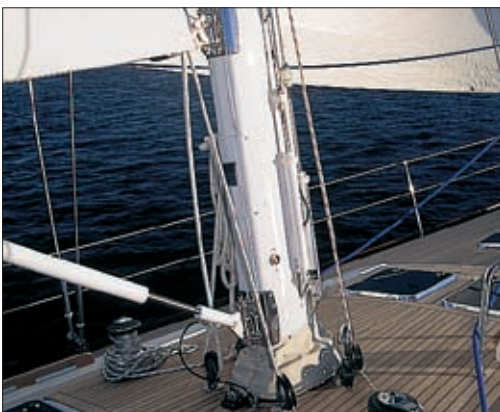
Rullmastens hydrauliska drivenhet ligger inkaplad i masten.
